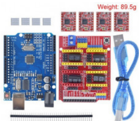
CNC Shield V3 + UNO R3 + 4*A4988+Cable
